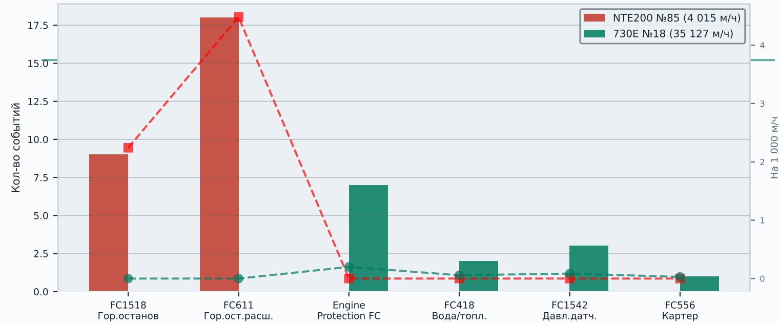
Сравнение FC-событий и защиты по данным INSITE KAMCC
